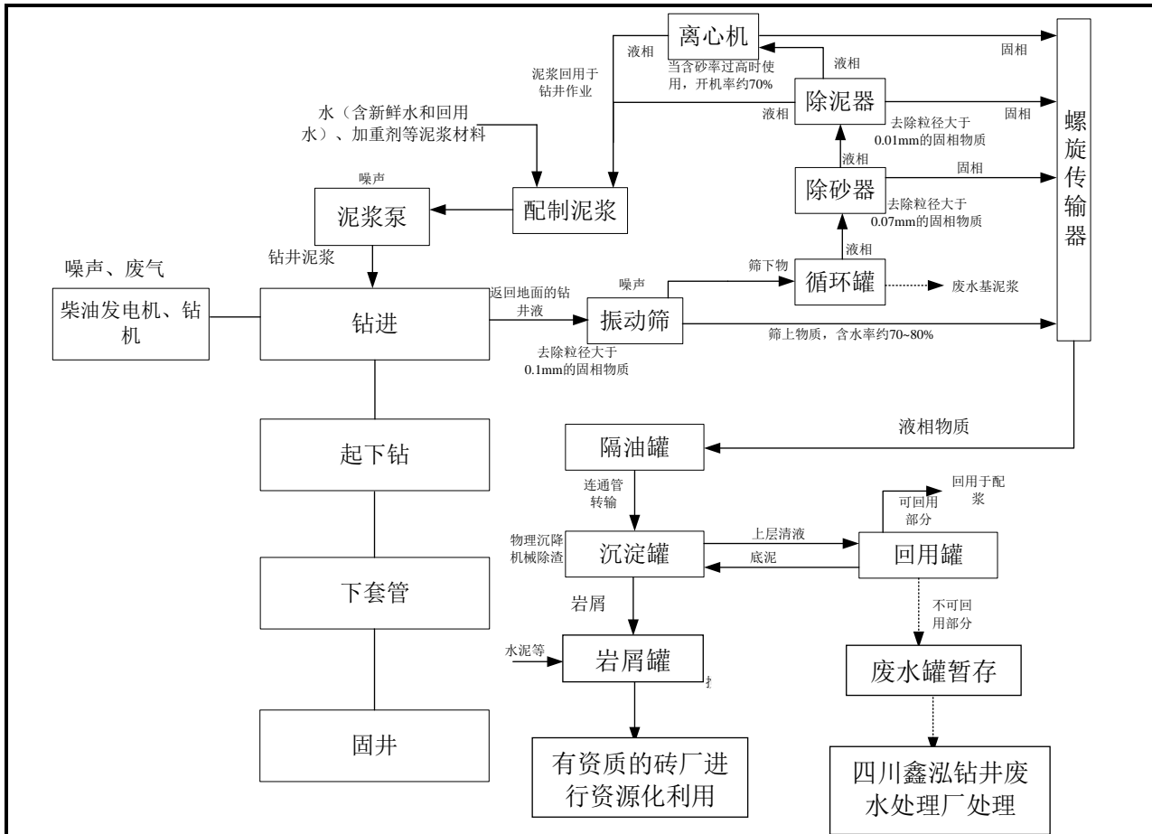
图 5.3-2 水基泥浆钻阶段作业流程及产污节点框图
