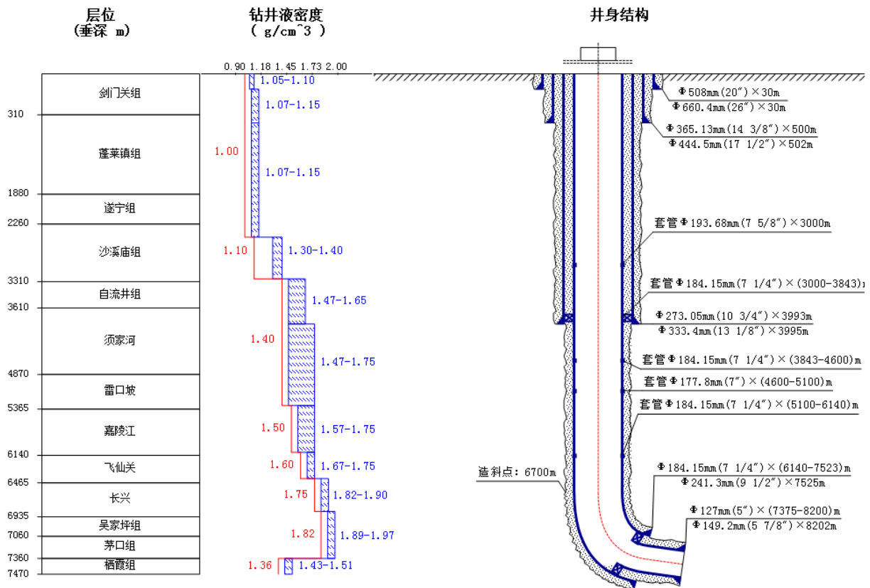
图 5.3-1 双鱼 001-X3 井钻井井身结构示意图
