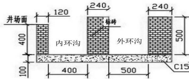
图 5.2-2 井场雨污分流排水沟结构图
