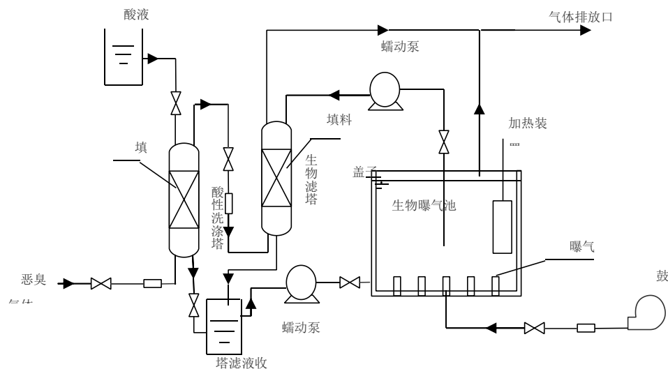
图 6-3 恶臭气体处理工艺流程图
