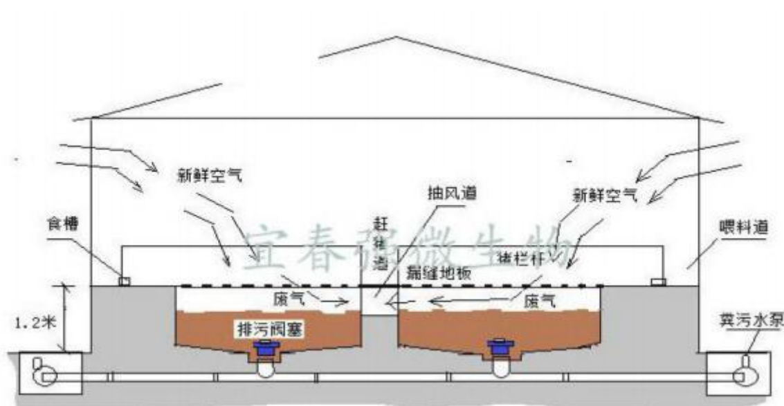
图 3-4 猪舍清粪工艺
