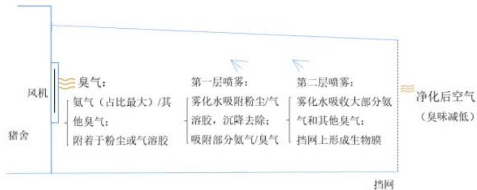
图 3-8 猪舍除臭装置示意图
