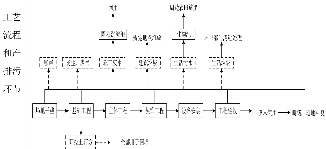
图 2-2 施工期工艺流程及产污位置图
