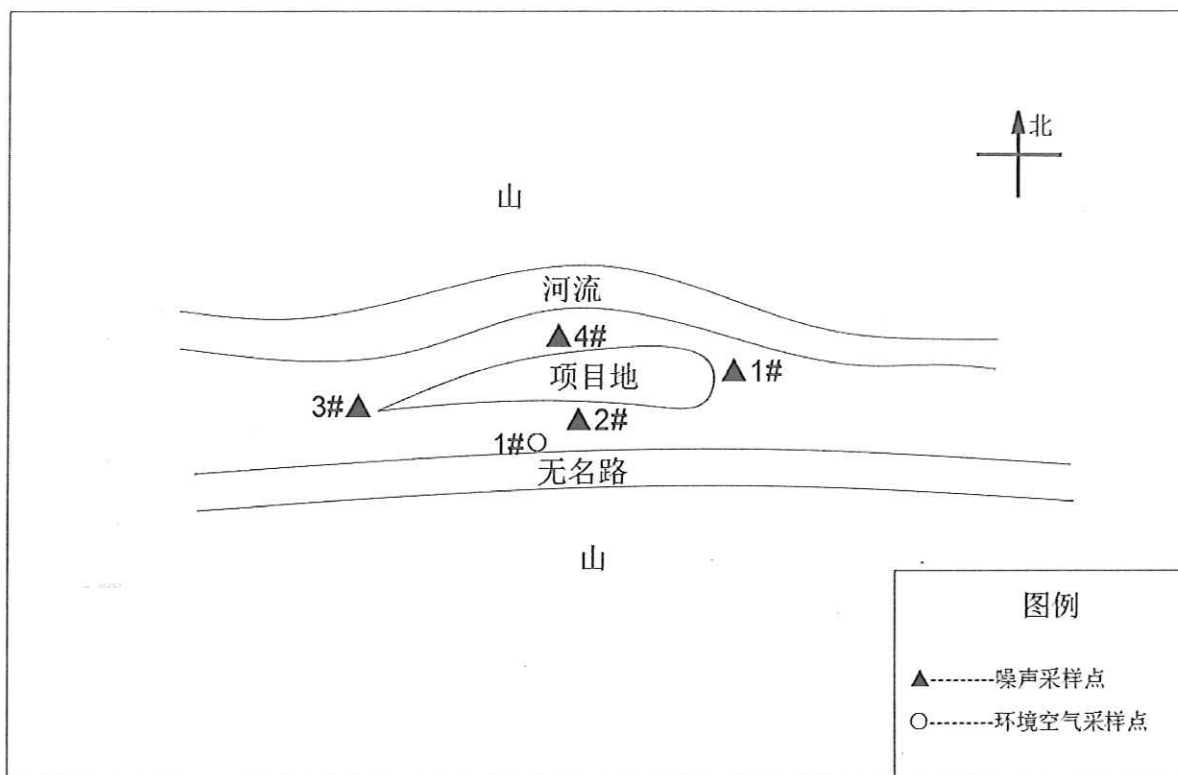
图 5-1 检测布点示意图
