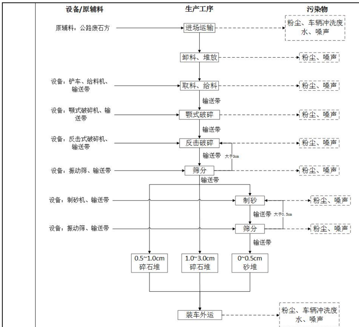
图2-3 项目生产加工工艺流程及产污环节图
