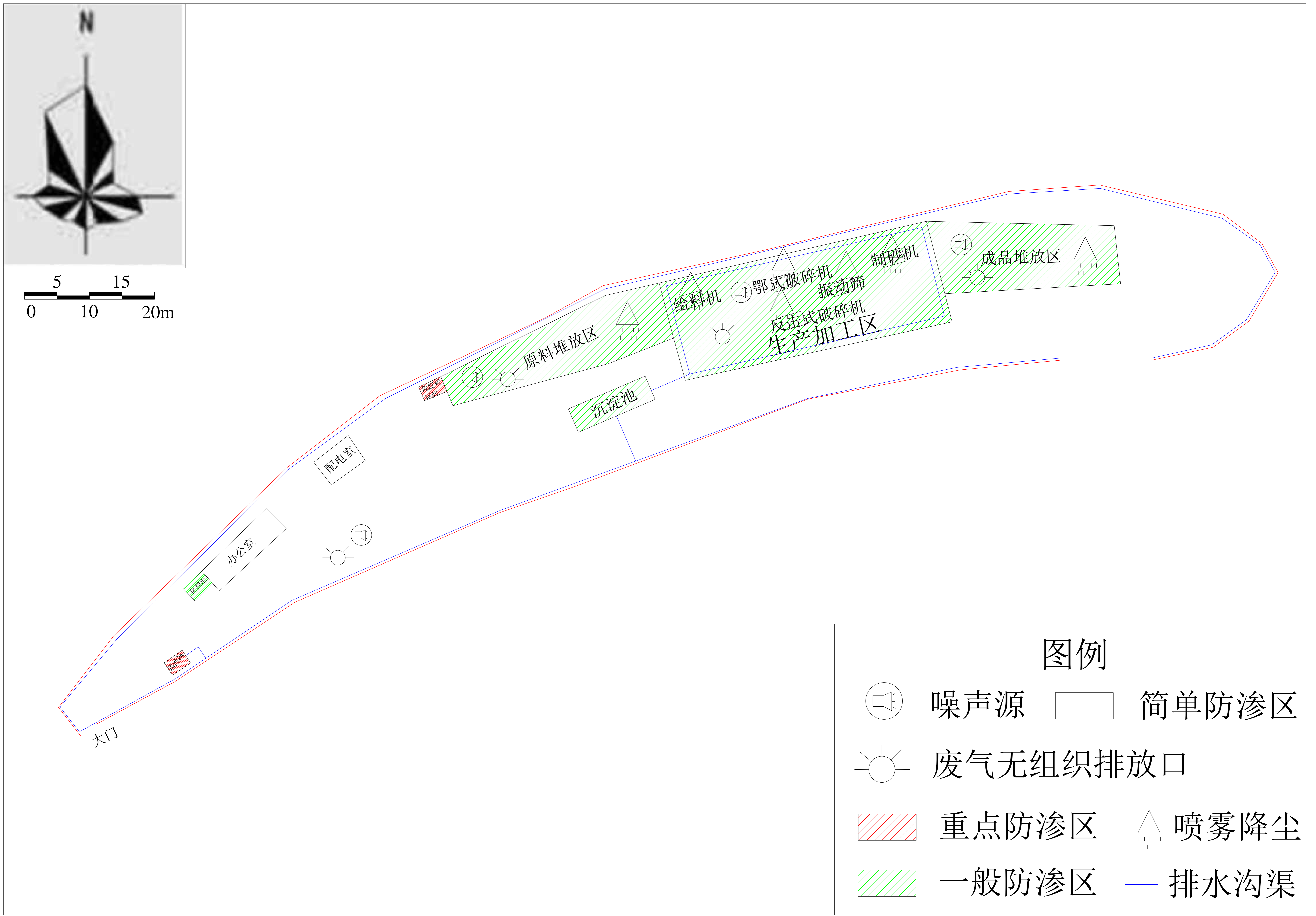
附图2 本项目总平面布置及分区防渗图
