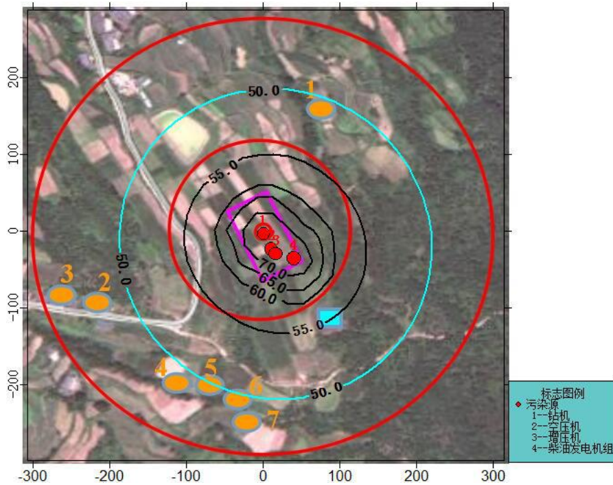
图 5.4-4 空气钻作业期间夜间噪声预测等声级图（声级单位：dB(A)）
