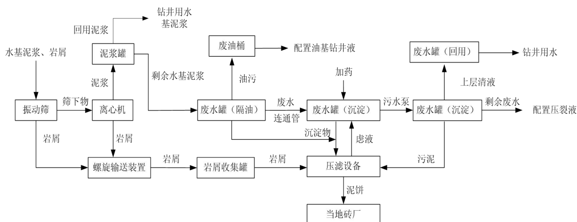
图 3.1-7 钻井现场清洁化生产方案处理流程示意图
