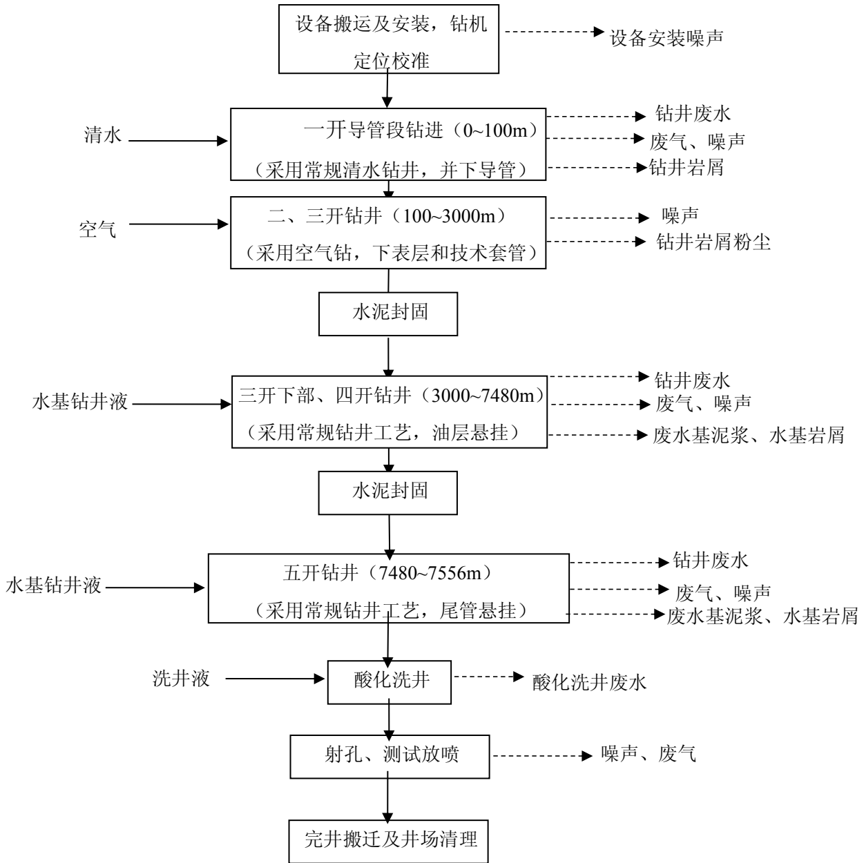
图 3.3-1 钻井作业工艺流程及产污节点示意图
