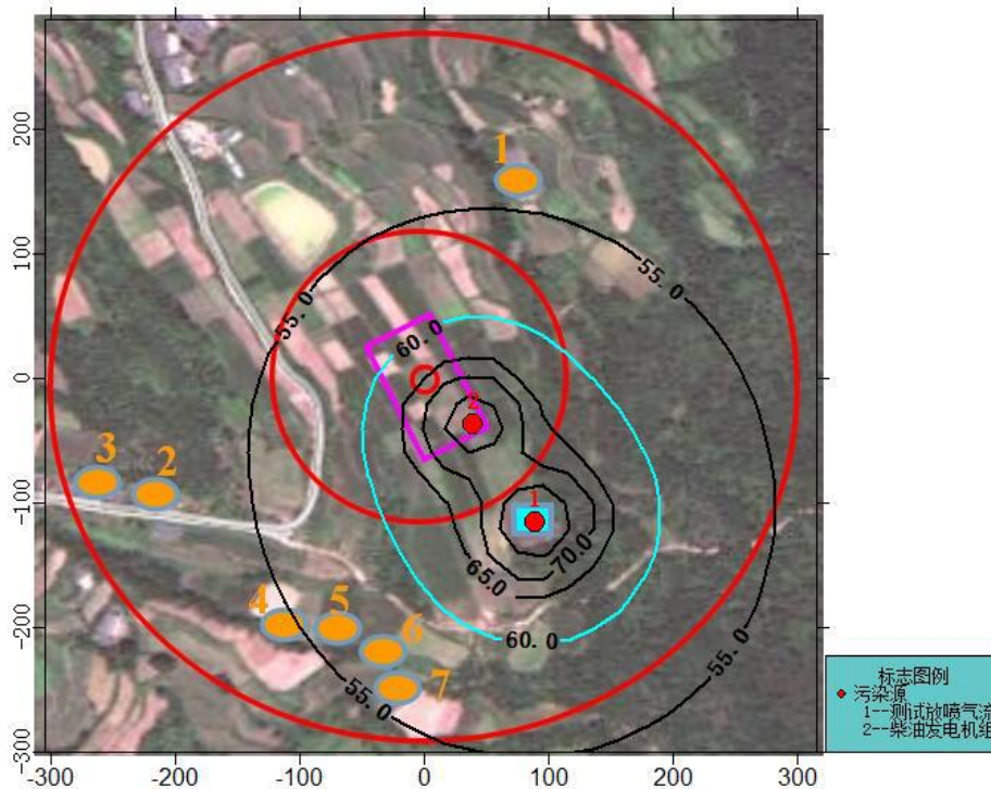
图 5.4-5 测试放喷作业期间噪声预测等声级图 (声级单位: dB(A))
