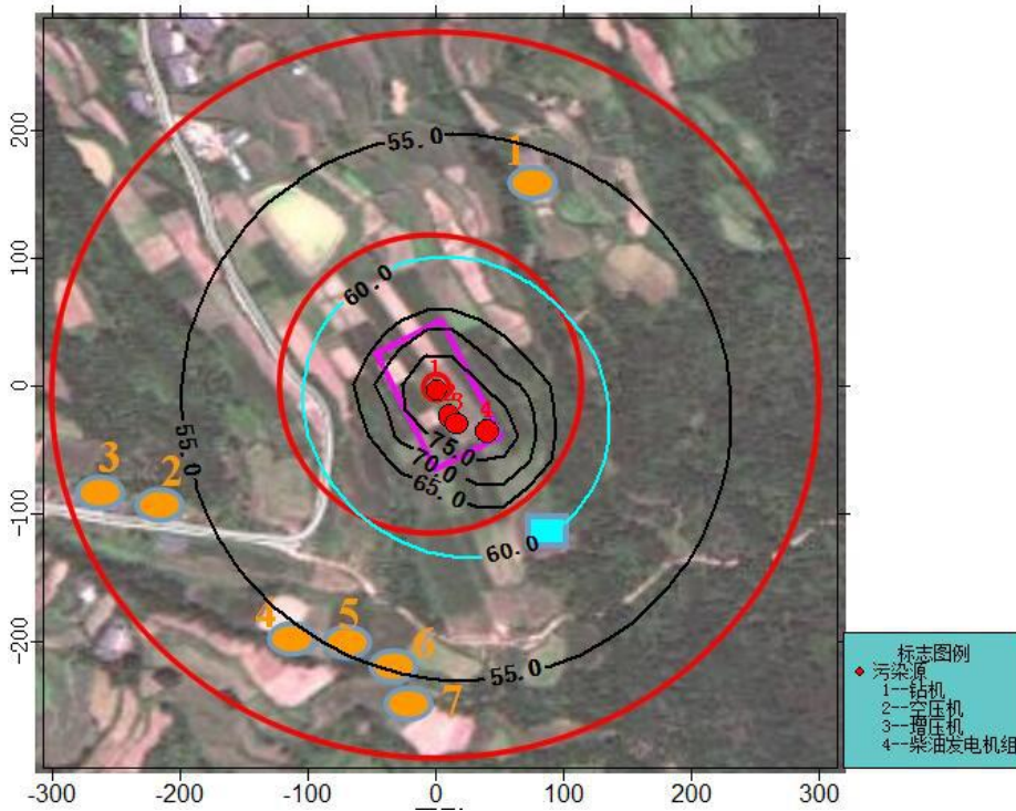
图 5.4-2 空气钻作业期间昼间噪声预测等声级图（声级单位：dB(A)）
