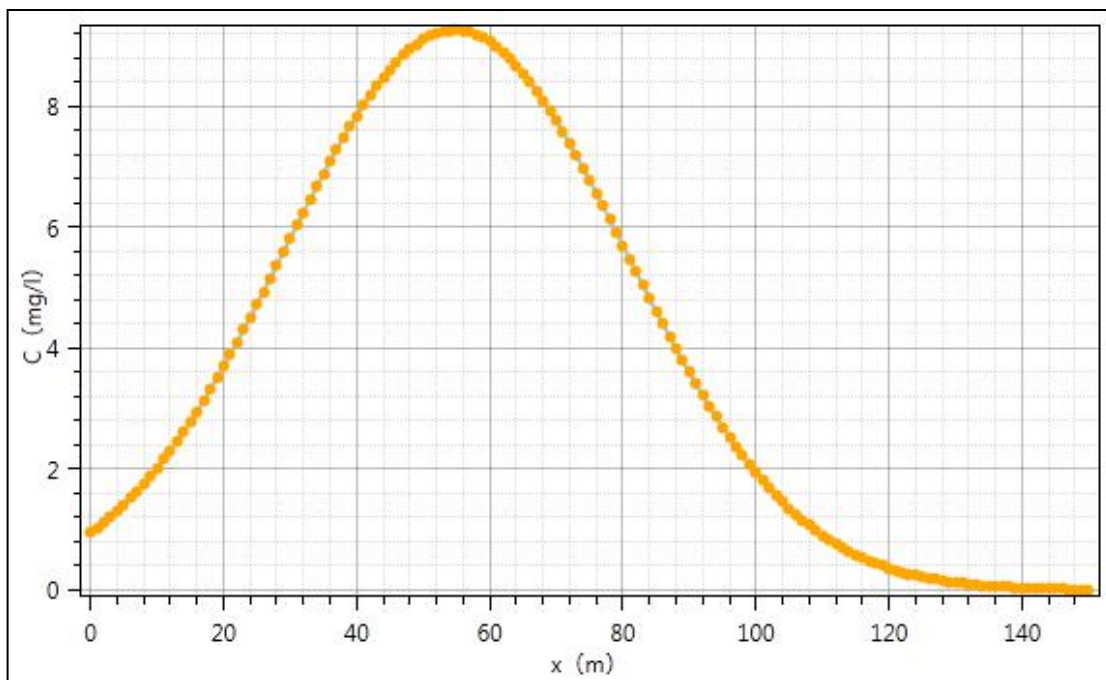
图 5.3-2 污染后 365 天水流下游轴向污染物总量浓度变化趋势图
