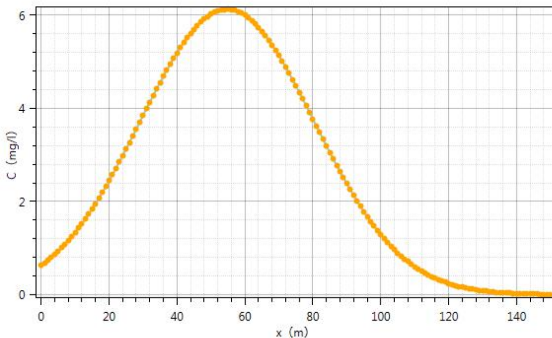
图 5.3-7 污染后 365 天水流下游轴向污染物总量浓度变化趋势图
