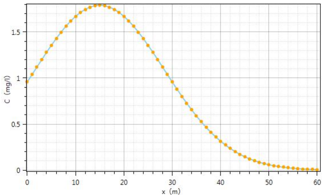
图 5.3-9 污染后 100 天水流下游轴向石油类浓度变化趋势图
