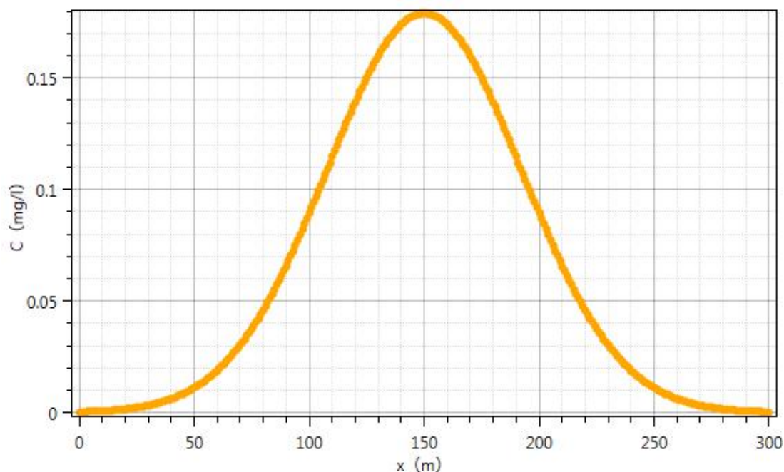
图 5.3-11 污染后 1000 天水流下游轴向石油类浓度变化趋势图
