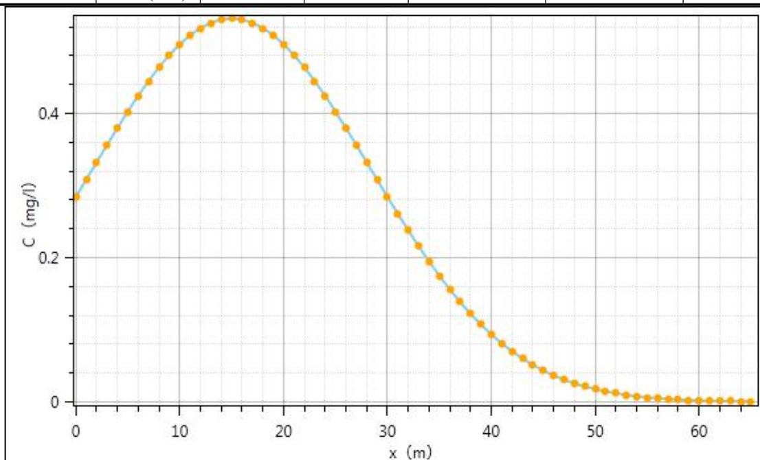
图 5.3-3 污染后 100 天水流下游轴向石油类浓度变化趋势图
