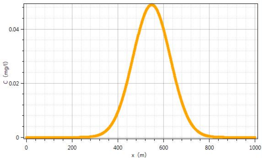
图 5.3-12 污染后 10a 天水流下游轴向石油类浓度变化趋势图
