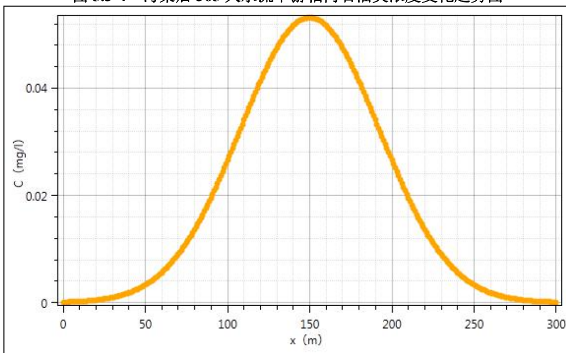
图 5.3-5 污染后 1000 天水流下游轴向石油类浓度变化趋势图
