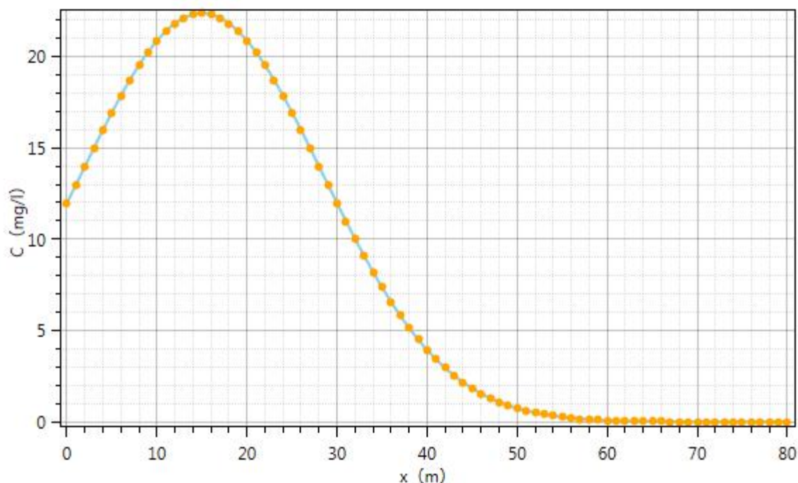
图 5.3-6 污染后 100 天水流下游轴向污染物总量浓度变化趋势图
