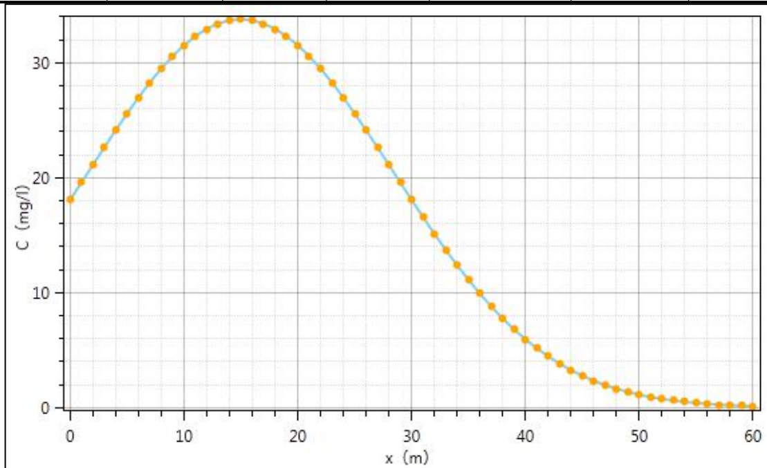
图 5.3-1 污染后 100 天水流下游轴向污染物总量浓度变化趋势图
