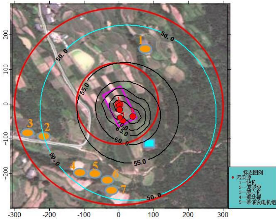
图 5.4-3 常规钻井作业期间夜间噪声预测等声级图（声级单位：dB(A)）
