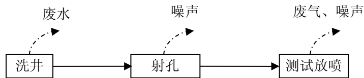
图 3.3-2 完井作业工艺流程及产污节点示意图
