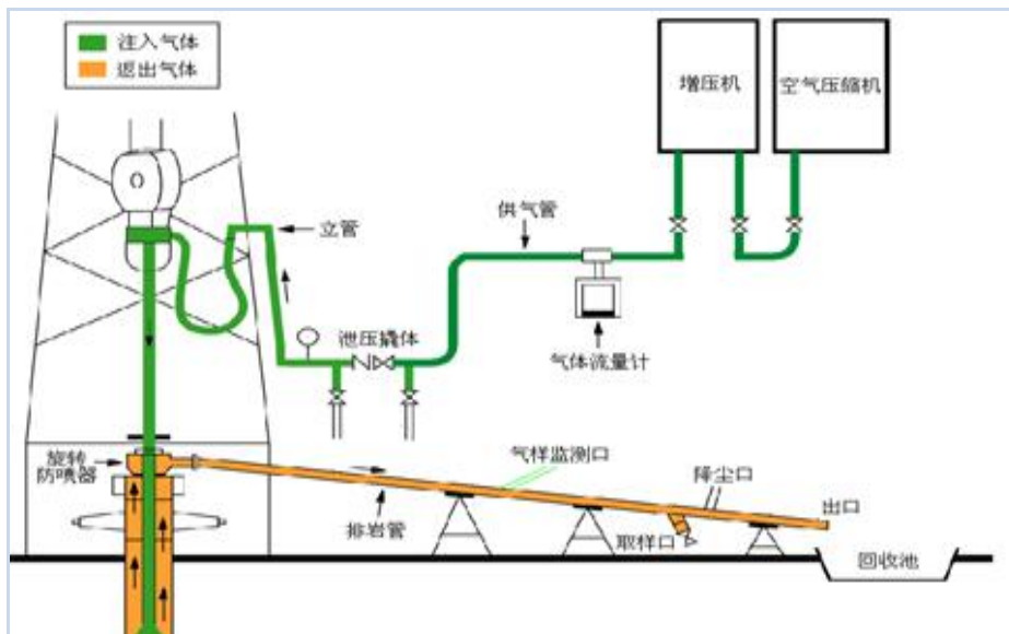
图 3.1-6 空气钻井工艺技术流程图
