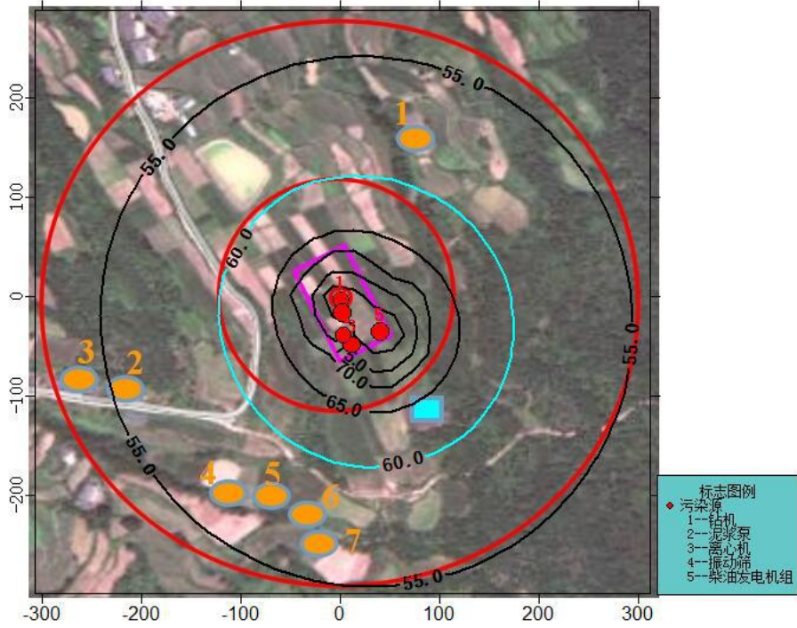
图 5.4-1 常规钻井作业期间昼间噪声预测等声级图（声级单位：dB(A)）
