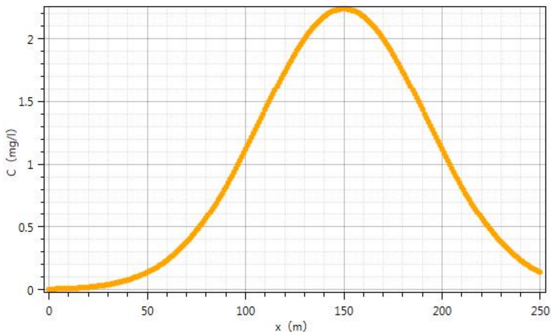
图 5.3-8 污染后 1000 天水流下游轴向污染物总量浓度变化趋势图
