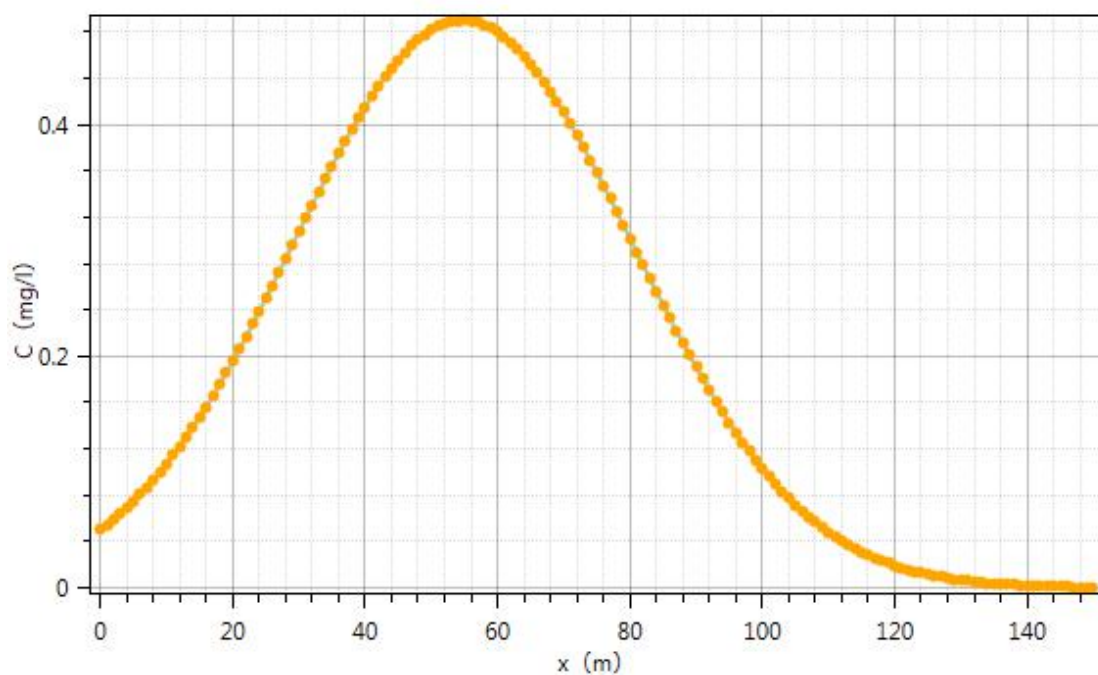
图 5.3-10 污染后 365 天水流下游轴向石油类浓度变化趋势图
