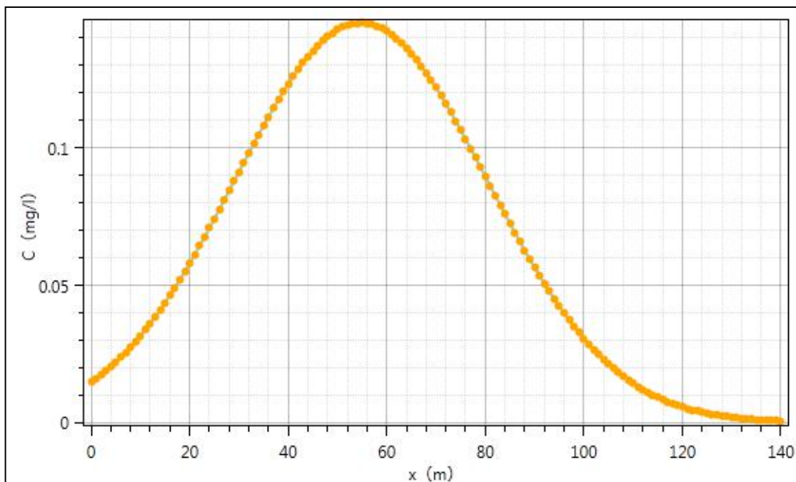
图 5.3-4 污染后 365 天水流下游轴向石油类浓度变化趋势图
