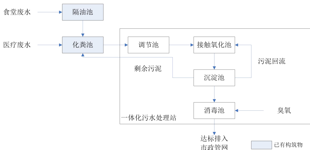
图4.2-4 项目污水处理工艺流程图
