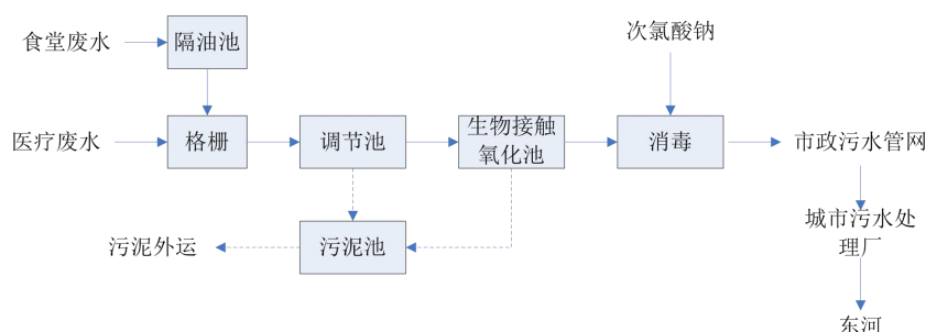
图 2.6-1 现污水处理站工艺流程图
