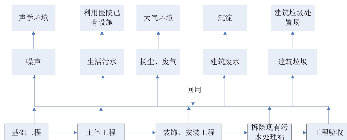
图 4.1-1 基础开挖、主体建筑物建设工艺流程及产污环节图
