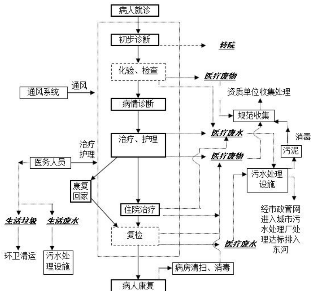
4.2-1 营运期工艺流程及产污环节图
