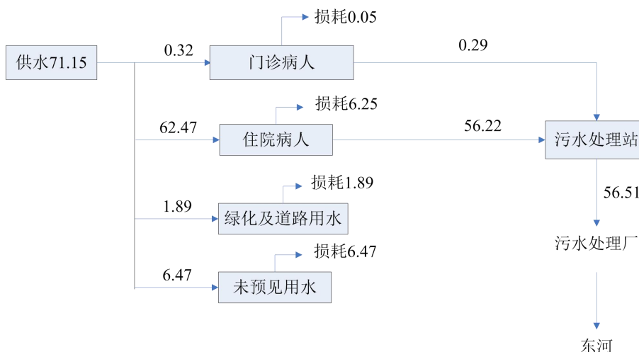
图4.2-2 本项目水平衡图（单位：t/d）
