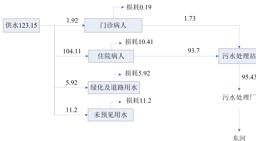
图4.2-3 建成后全院水平衡图（单位：t/d）
